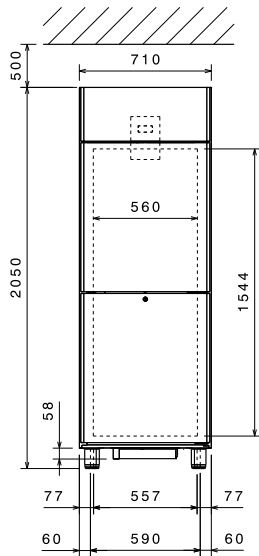
Front aanzicht
